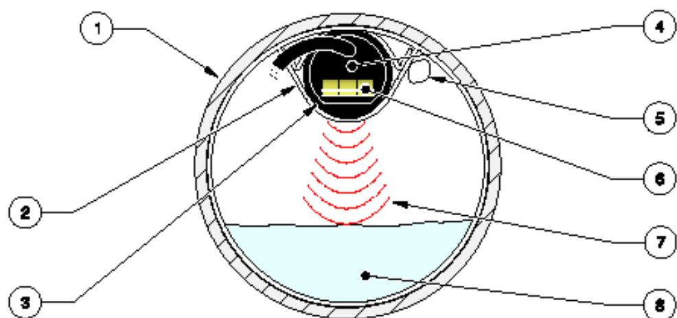
图 37 管道端视图
