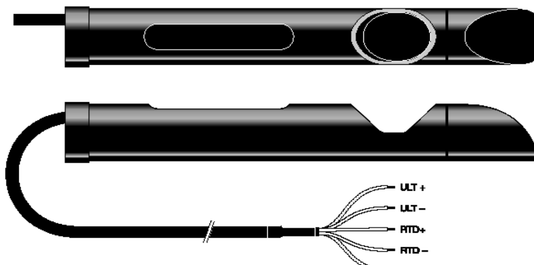
图 24 管道内超声波传感器
