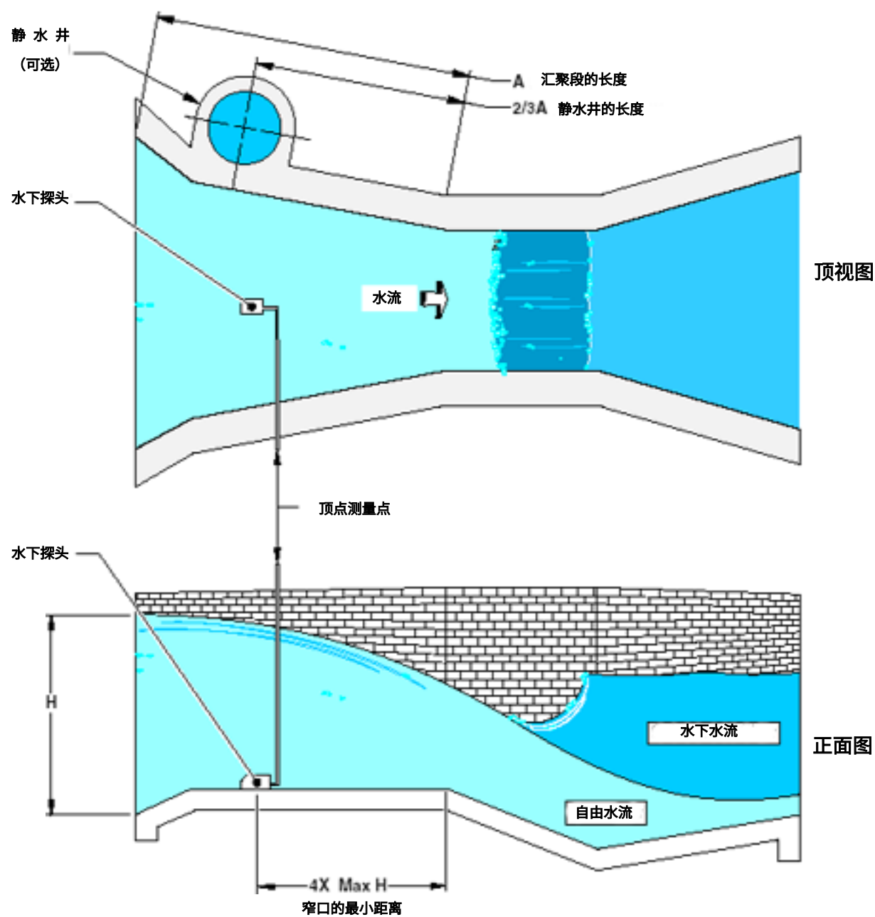
图 51 Parshall 型水槽
