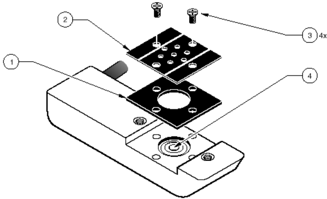
图 47 移开保护盖
