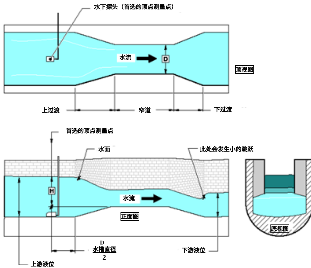
图 53 Leopold-Lagco 型水槽
