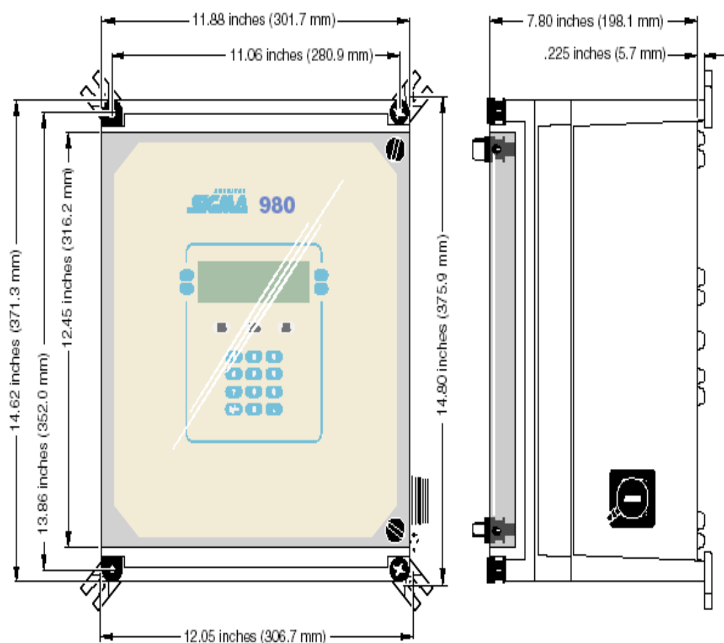
图 5 安装尺寸 (1)
