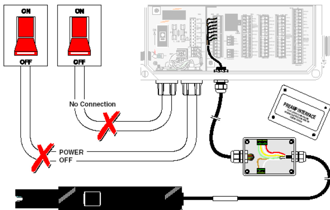
图 21 仪器接线盒
