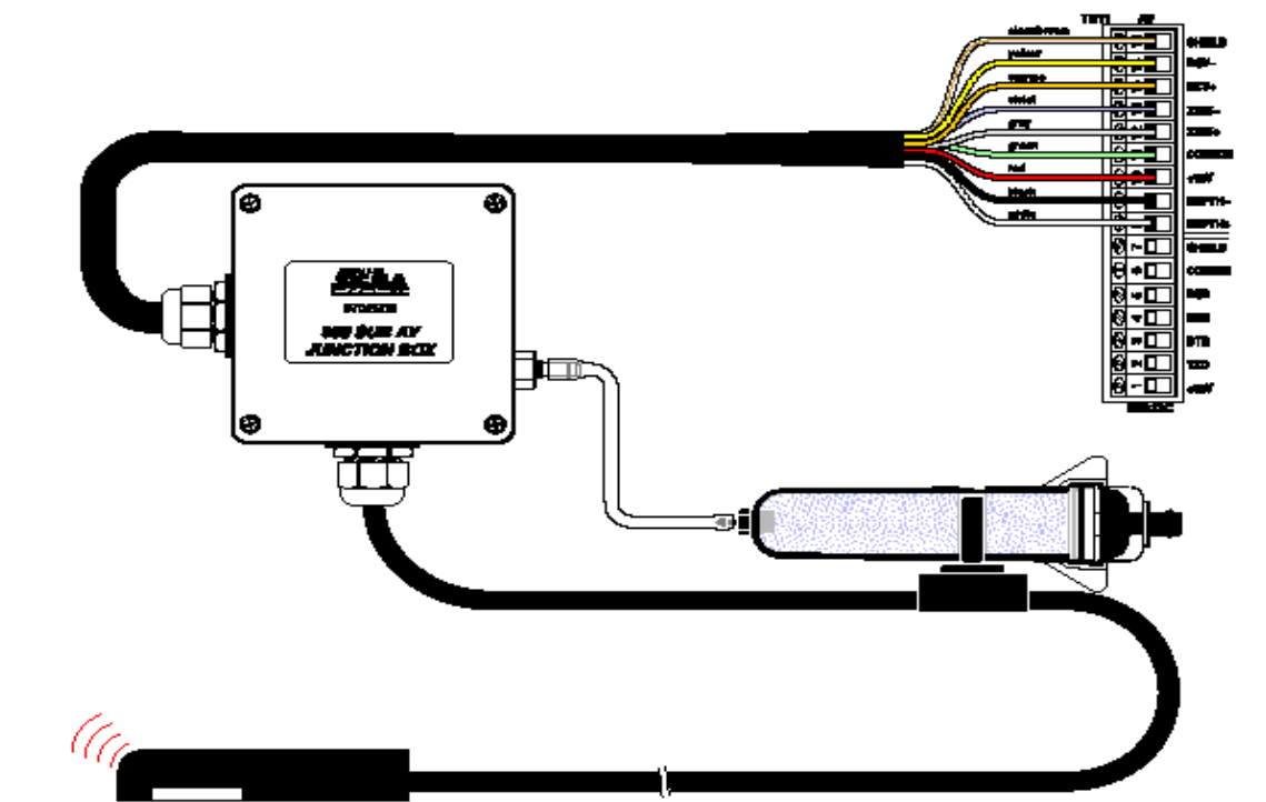
图 27 接线盒，探头，线缆连接和干燥管
