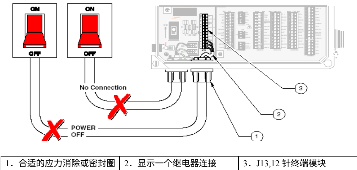
图 16 警报继电器 TB13 的定位
