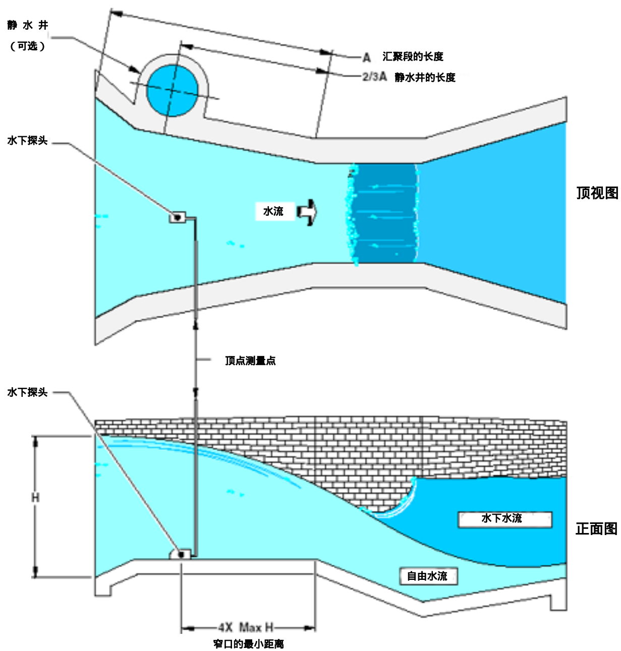
图 51 Parshall 型水槽
